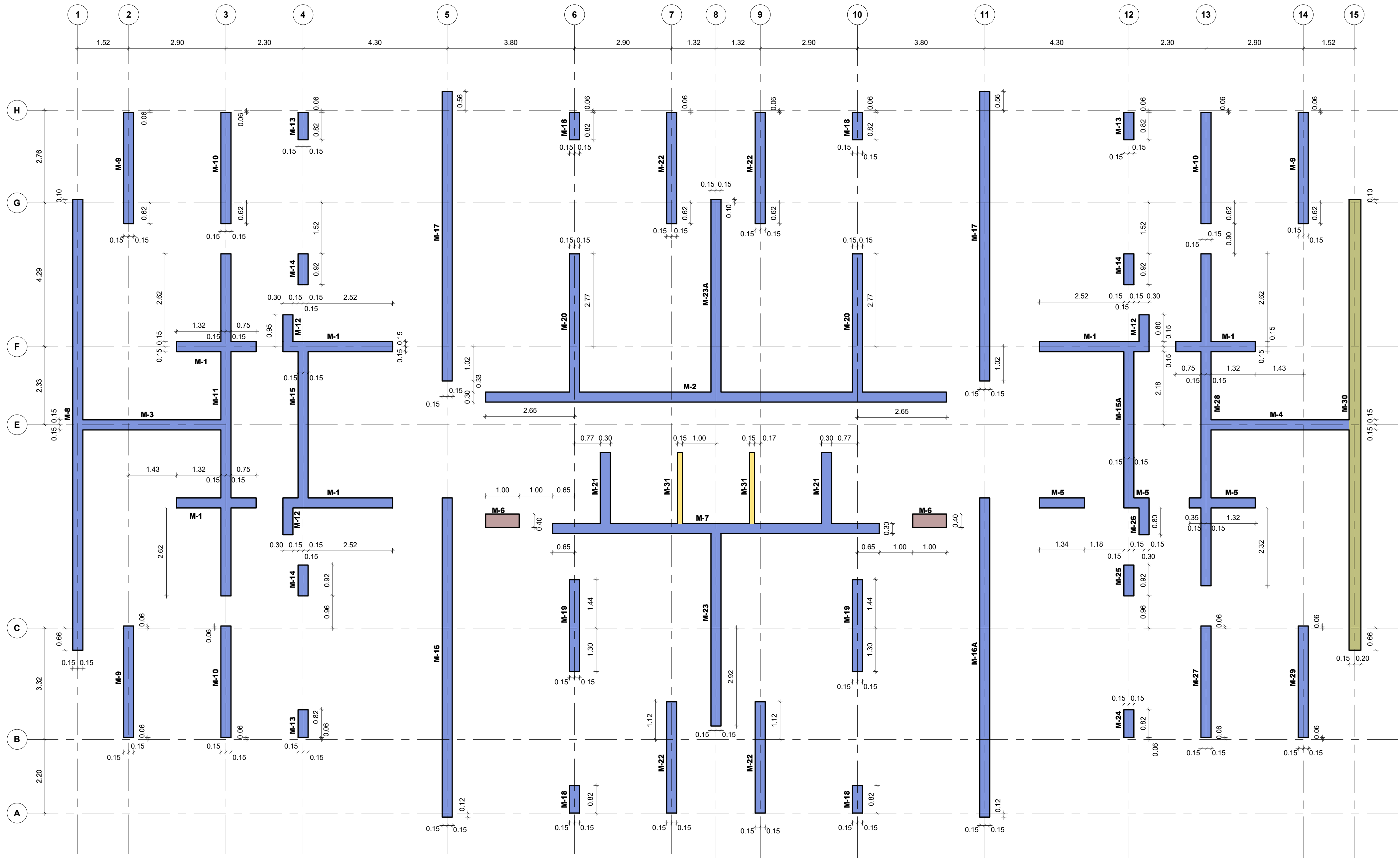
PLANTA LOCALIZACIÓN DE MUROS PISO 1 Escala 1 : 75
